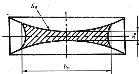
图 9 矩形横截面试样缩颈处最大宽度和最小厚度
