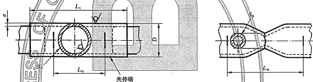
图 13 管的纵向弧形试样(见附录 D)
