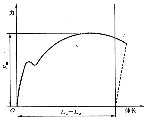
图 8 最大力( F_m )
