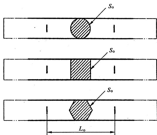
图 11 比例试样(见附录 B)
