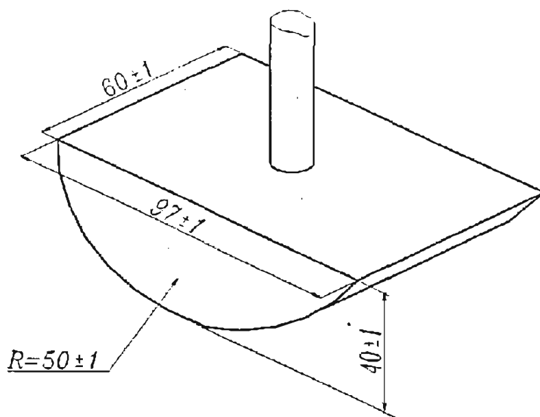
图 E.1 横向变形试验测试头
