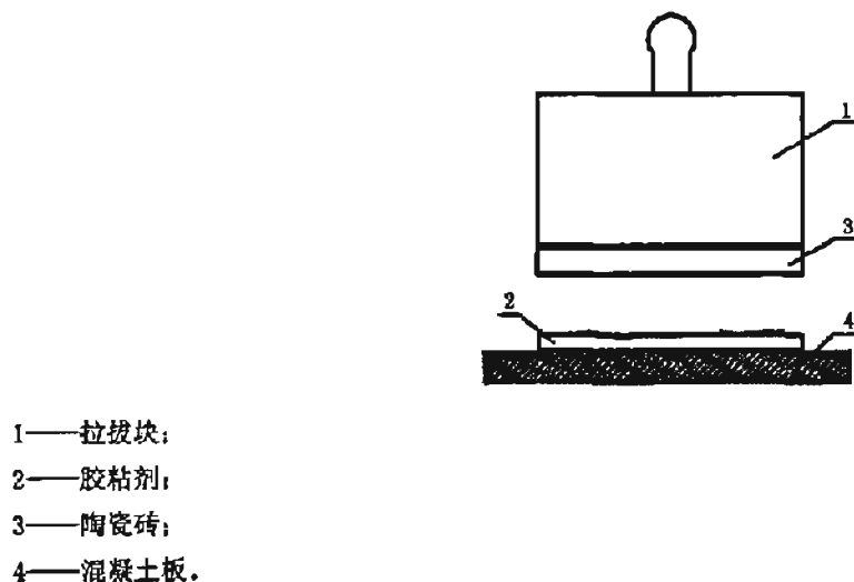
图 B.2 发生在陶瓷砖和胶粘剂层界面(AF—T)的破坏
