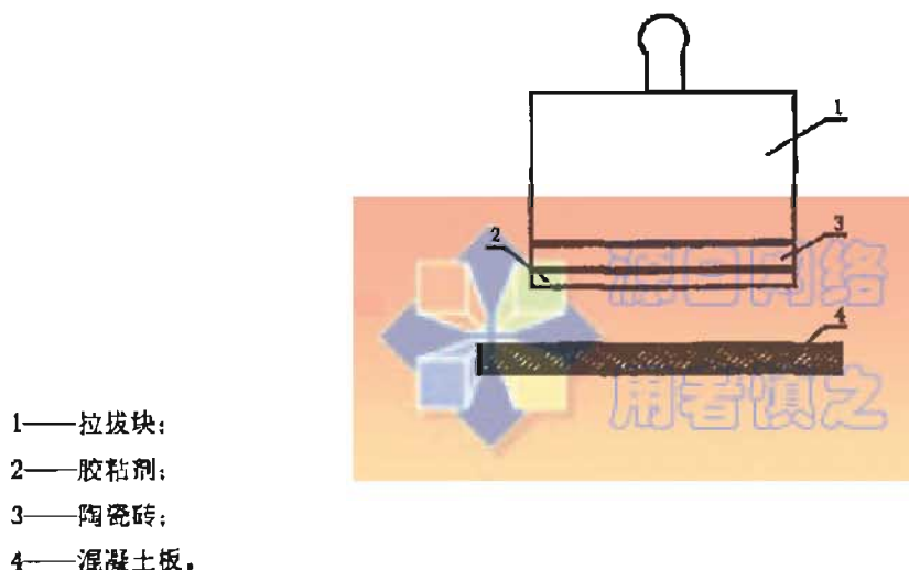
图 B.1 发生在胶粘剂层和基材的界面(AF—S)的破坏
