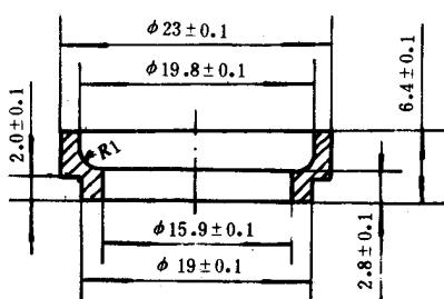
a 黄铜肩环
