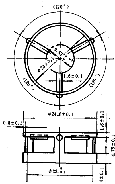
图3 钢球定位环
