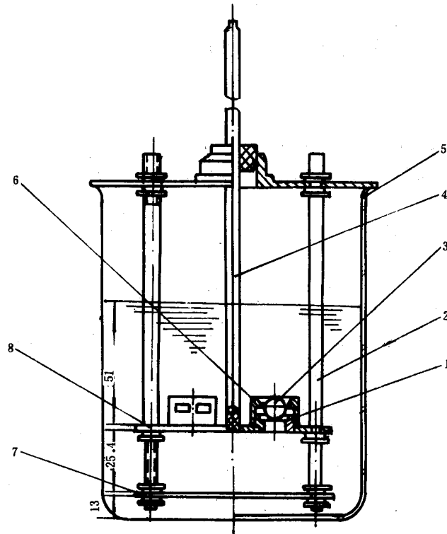
图 1 软化点测定器装置
