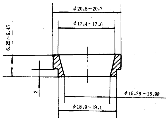
b 黄铜锥环
