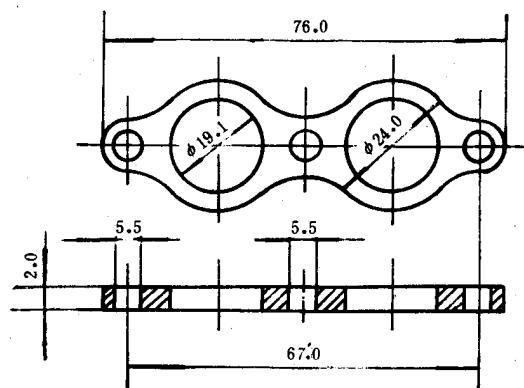
图 2 环架金属板
